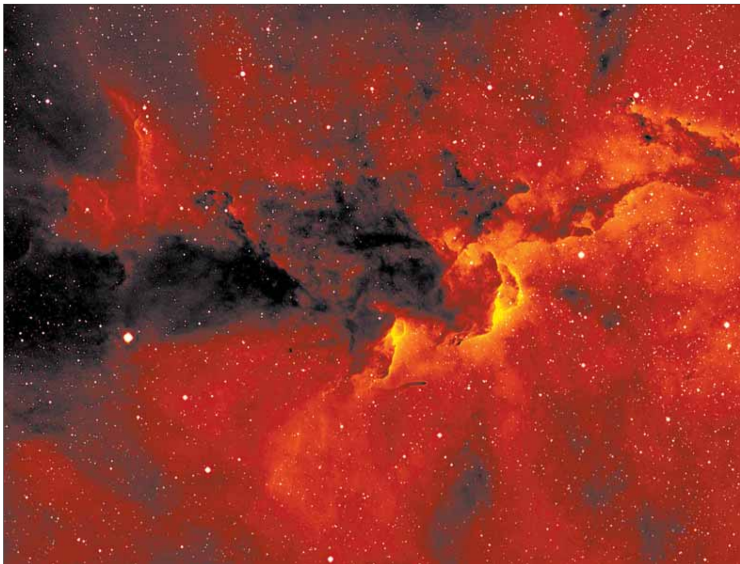
Imagen de la Nebulosa Trompa de Elefante, tomada por el telescopio Isaac Newton de la Isla de la Palma, para el proyecto IPHAS Survey.
